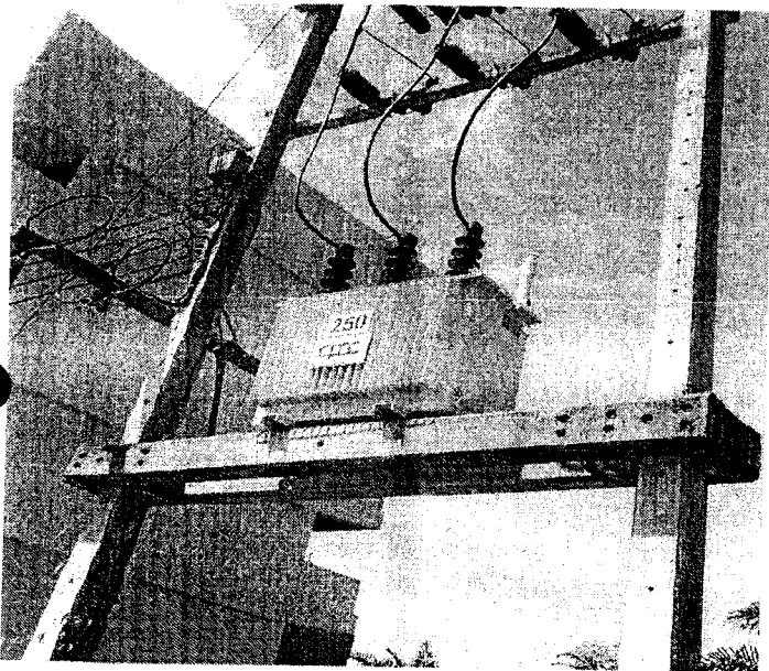
11.หม้อแปลงอาคารแฟลต 32 ยูนิต 250kva
