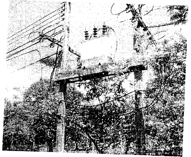
1.หม้อแปลงประปาหน้ามหาวิทยาลัย 100kva 2.หม้อแปลงอาคารสำนักงานวิทยาเขต 250 kva
